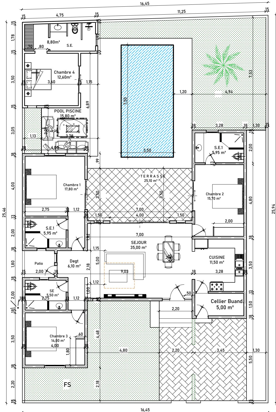
PLAN LOT 27 (B) Terrain = 422,50 m 2 Surface Bâtie: 166,50 m 2 Annexe : 37,30 m 2
